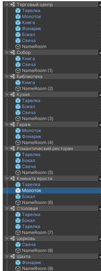
Рисунок 40 – Заполнение базы
