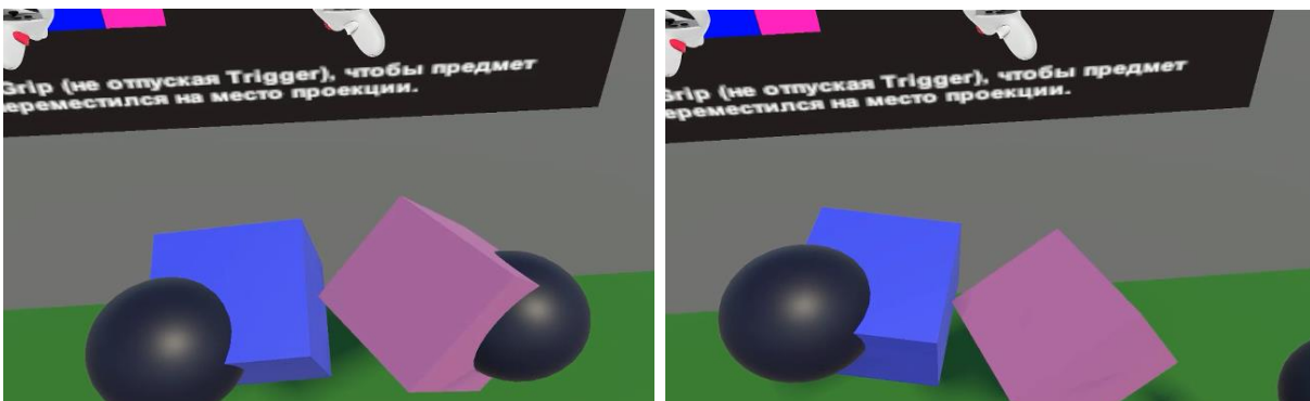
Рисунок 34 – Соединение объектов
