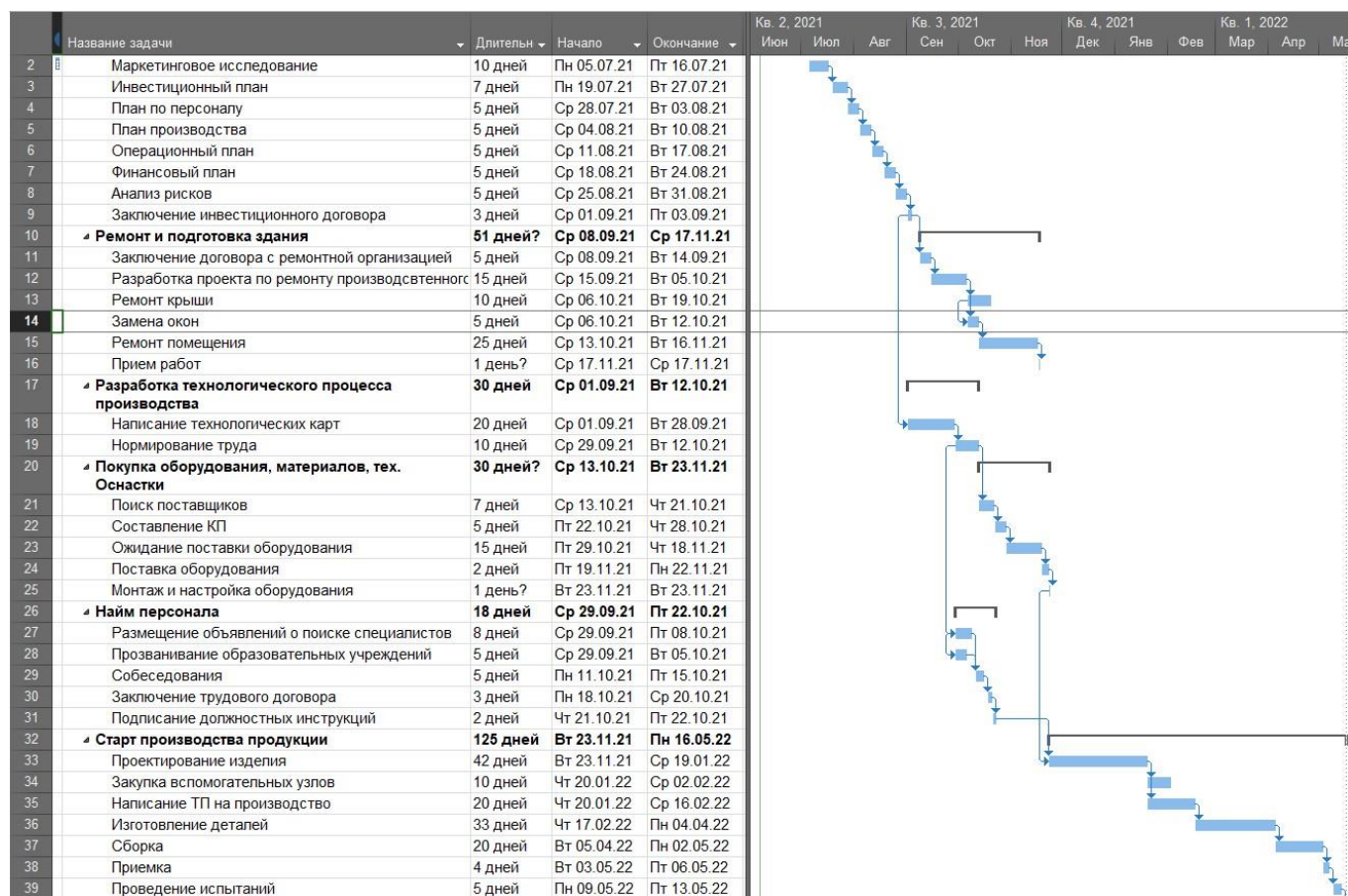
Рисунок 3.1 – Диаграмма Ганта
